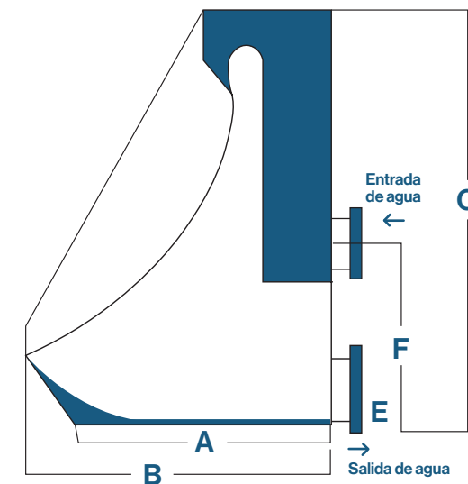
CORTE LATERAL
